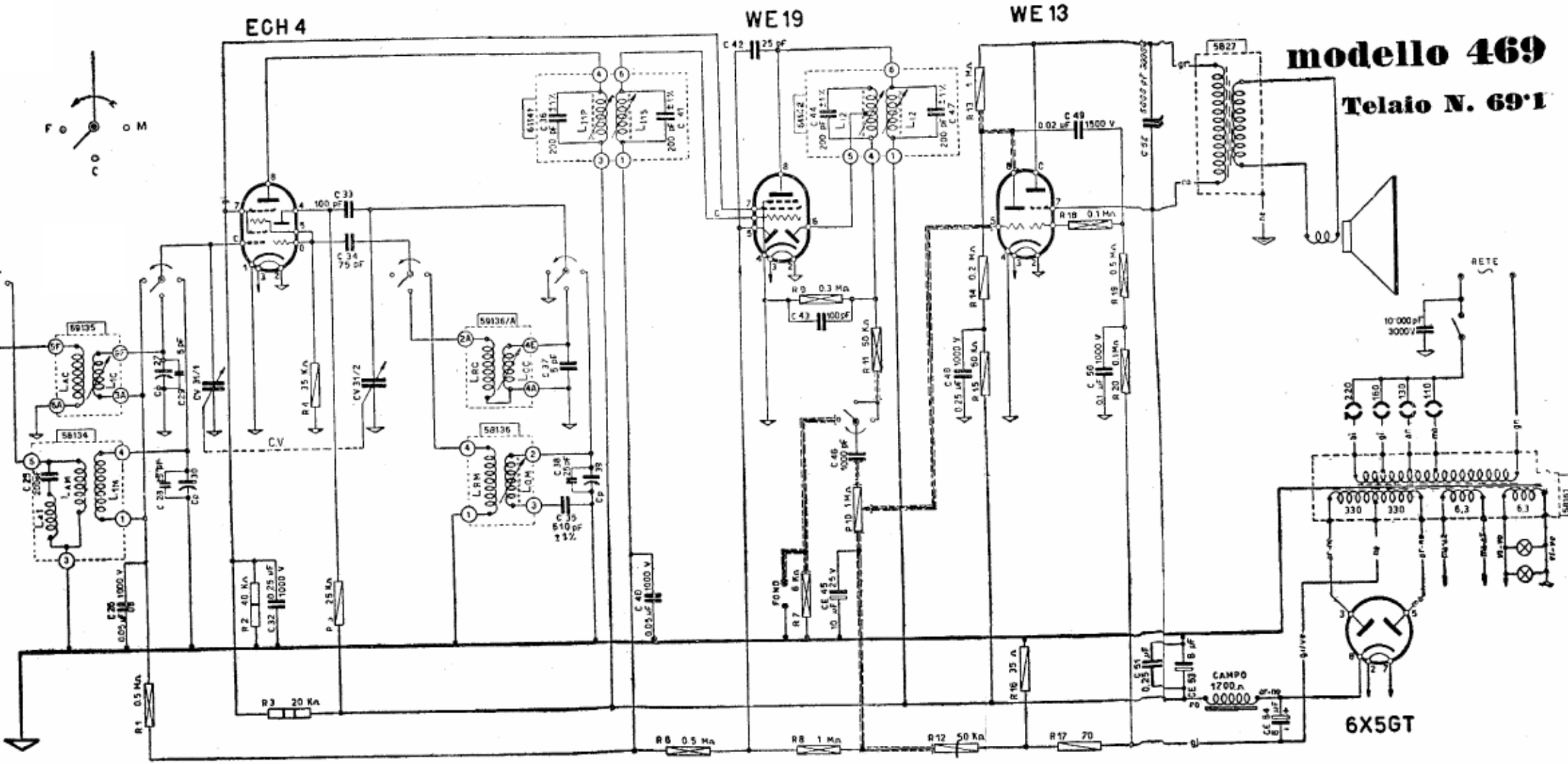
LA VOCE DEL PADRONE. — Mod. 469 e 478. — Telaio 69.1. — Produzione 1941. — Due gamme d'onde: onde medie 190 e 580 m; onde corte 15 a 52 m. — Media frequenza: 465 kHz. Stesso schema anche per il mod. 458 con ECH3.
